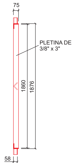
SECCION B-B
