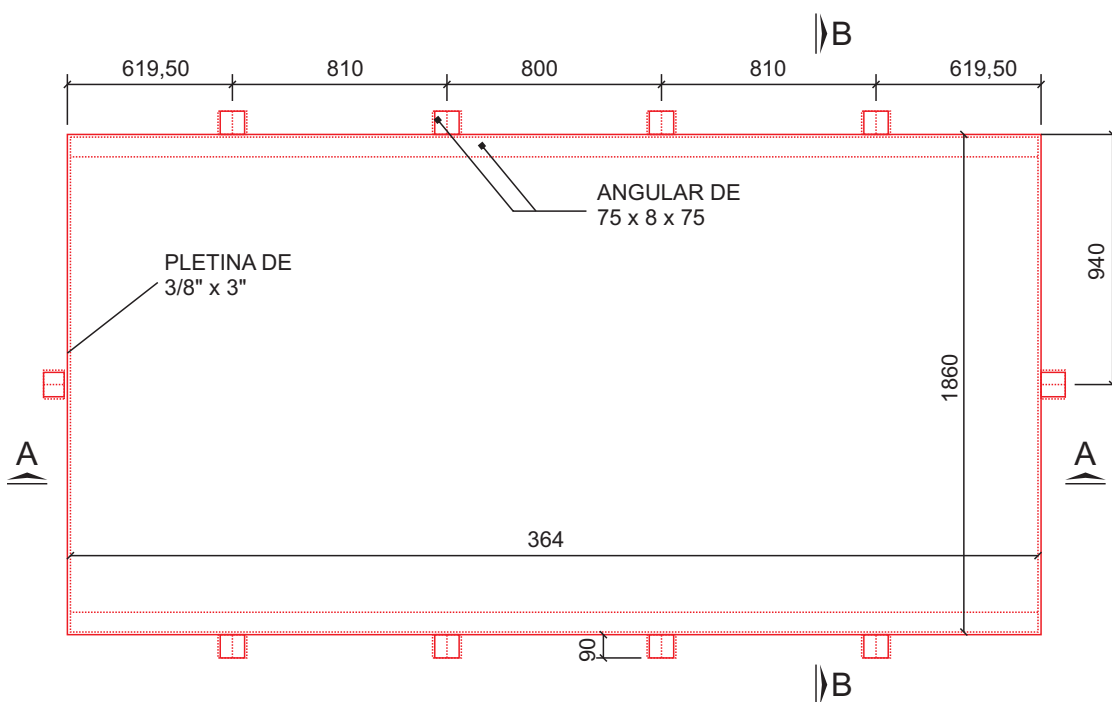
PLANTA
