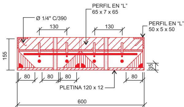
SECCION B-B
