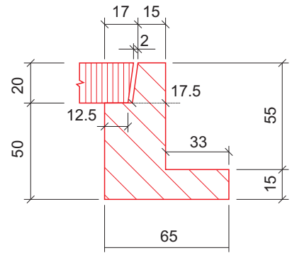
SECCION DETALLE MARCO
