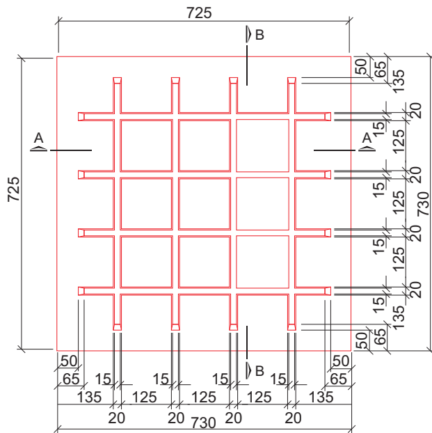
VISTA INFERIOR TAPA
