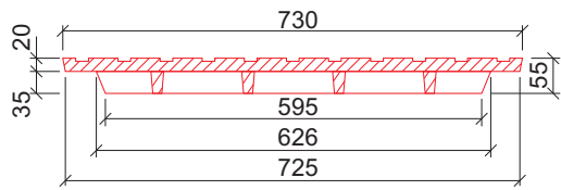
SECCION A-A
