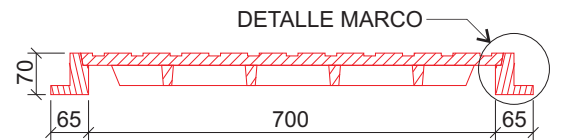
SECCION C-C
