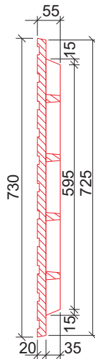
SECCION B-B
